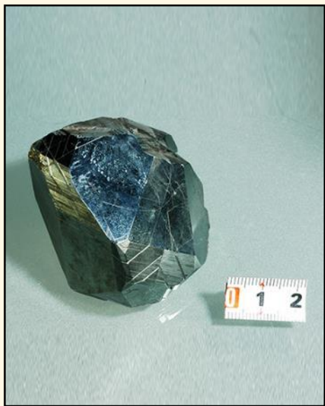
赤鐵礦
