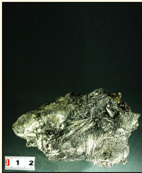
硫銻鉛礦
